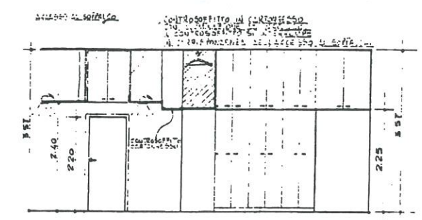
SEZIONE X-Y
